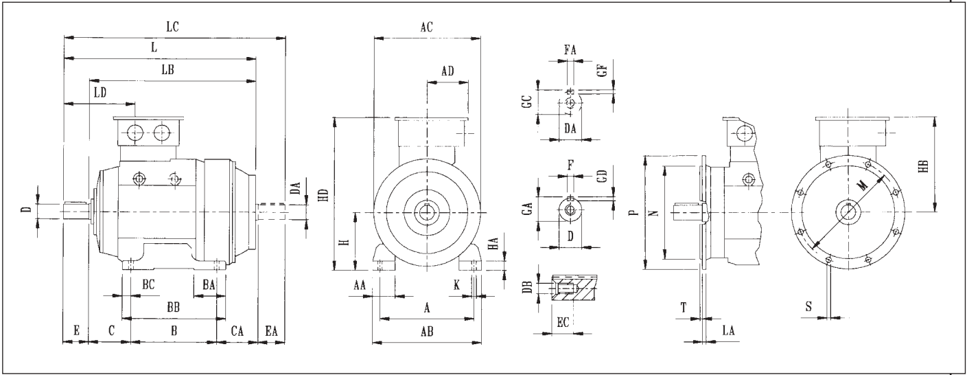
Coupling dimensions
